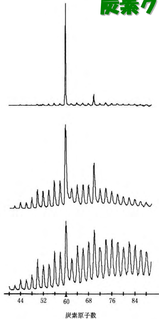
図 2.4 C_{60} の強い magic number 性が観測された、炭素クラスターの質量スペクトル。下の図と中の図はそれぞれヘリウムの圧力が 10 Torr と 760 Torr, 上の図はヘリウム圧が 760 Torr でノズルの先端にクラスター成長管をつけた場合 7) 。
