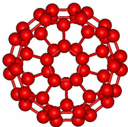
C_{60} - I_h
