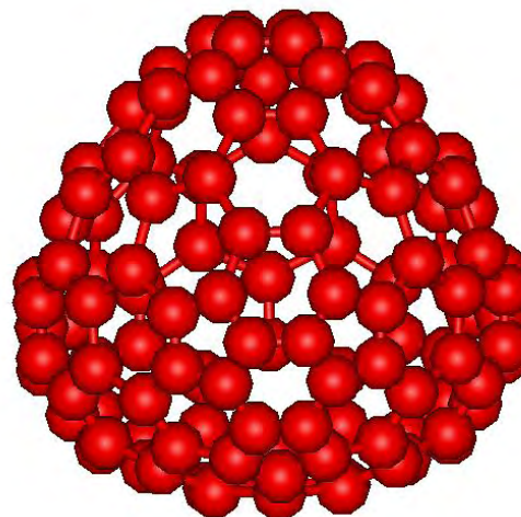
C_{120} - T_d
