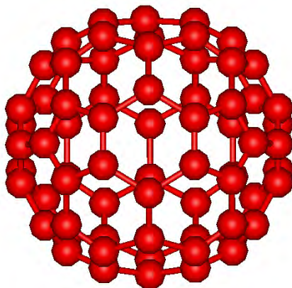
C_{70} - D_{5h}
